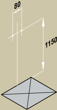
Cotas conexión de fontanería / Plumbing connections
