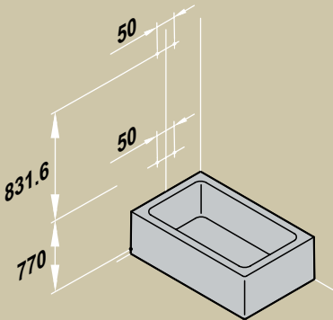
Cotas conexión de fontanería / Plumbing connections
