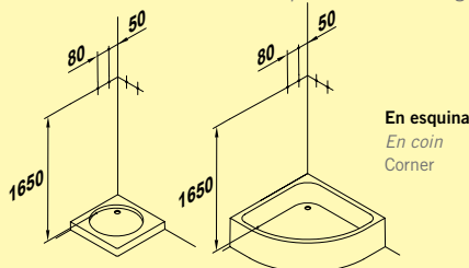
Cotas conexiones fontanería Cotes connexions plomberie Plumbing connections
