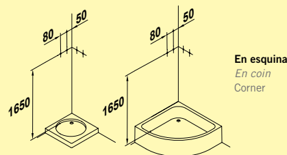
Cotas conexiones fontanería Cotes connexions plomberie Plumbing connections
