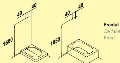
Cotas conexiones fontanería Cotes connexions plomberie Plumbing connections
