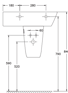
31433 Semipedestal Pop (orificio izquierda). Con juego de fijación. Para instalación en lavabos con orificio de grifería, situado en la parte izquierda.
