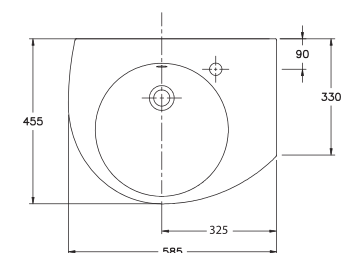
31050 Lavabo Pop de 58,5 x 45,5 cm. Asimétrico cubeta izquierda. Con rebosadero y juego de fijación. Válido para mural, semipedestal o sobre-encimera.
