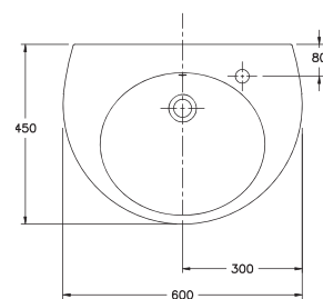
31010 Lavabo Pop de 60 x 45 cm. Con rebosadero y juego de fijación. Válido para mural, semipedestal o sobre-encimera.
