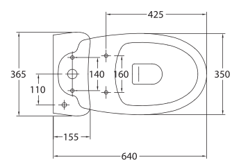
31180 Inodoro de 64 x 35 cm. salida horizontal. con juego anclaje.
