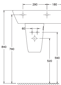
31432 Semipedestal Pop (orificio derecha). Con juego de fijación. Para instalación en lavabos con orificio de grifería, situado en la parte derecha.
