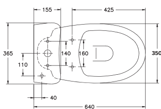
31150 Inodoro de 64 x 35 cm. salida vertical. con juego de anclaje.
