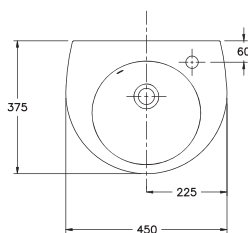
31080 Lavamanos Pop 45 x 37,5 cm. Con rebosadero y juego de fijación. Válido para mural o sobre-encimera.
