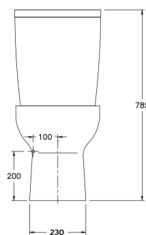
31150 Inodoro de 64 x 35 cm. salida vertical. con juego de anclaje.
