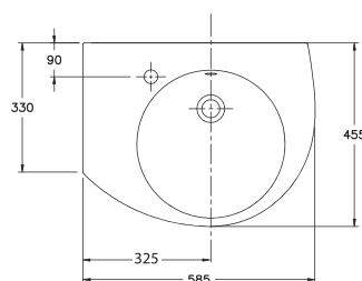
31040 Lavabo Pop de 58,5 x 45,5 cm. Asimétrico cubeta derecha. Con rebosadero y juego de fijación. Válido para mural, semipedestal o sobre-encimera.
