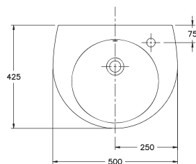
31030 Lavabo Pop de 50 x 42,5 cm. Con rebosadero y juego de fijación. Válido para mural, semipedestal o sobre-encimera.
