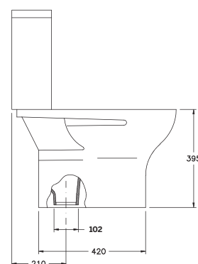
31540 Tanque bajo con tapa y mecanismo de doble pulsador. Alimentación inferior izquierda.
