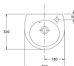
31090 Lavamanos Pop 36 x 32 cm. Con rebosadero y juego de fijación. Válido para mural o sobre-encimera.
