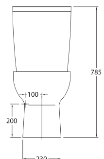
31180 Inodoro de 64 x 35 cm. salida horizontal. con juego anclaje.
