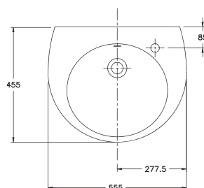
31020 Lavabo Pop de 55,5 x 45,5 cm. Con rebosadero y juego de fijación. Válido para mural, semipedestal o sobre-encimera.
