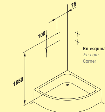
Cotas conexiones fontanería Cotes connexions plomberie Plumbing connections
