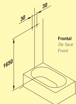
Cotas conexiones fontanería Cotes connexions plomberie Plumbing connections
