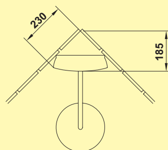
En esquina En coin Corner
