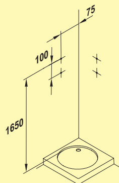
Cotas conexiones fontanería Cotes connexions plomberie Plumbing connections
