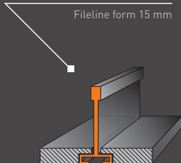
Perfil fineline de 15 mm Fileline form 15 mm
