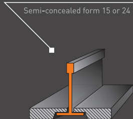
Perfil semioculto de 15 ó 24 mm Semi-concealed form 15 or 24 mm
