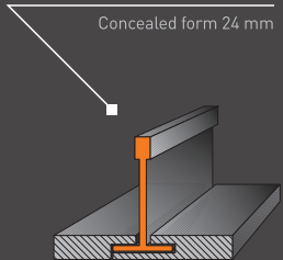
Perfil oculto de 24 mm Concealed form 24 mm
