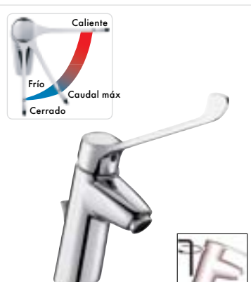
E18161 Monomando lavabo Easy. Con cartucho secuencial y palanca larga. Vaciador automático. Fijación rápida por arriba.
