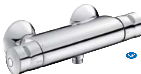
E71070 Grifería termostática de ducha mural, racores murales. Economizador de agua. Tope de seguridad a 38°C. Válvulas anti-retorno integradas en el cuerpo de la grifería.
