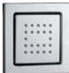
E8003 WaterTile Square Ducha lateral, 22 salidas. Medidas: 124x124x6 mm. Caudal max: 9,5 l/min.
