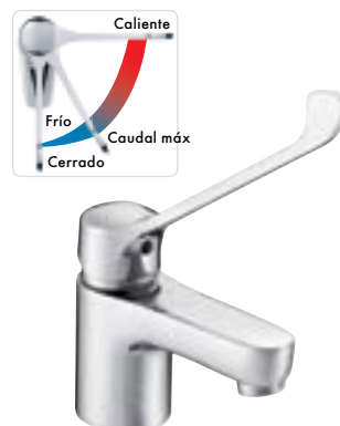
E16024-4 Monomando lavabo July Easy con palanca de 150 mm Vaciador automático, cartucho secuencial pre-regulado a 40° C de temperatura.
