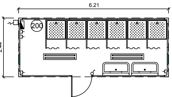
MÓDULO SANIT 15 M² (4L 6D)
