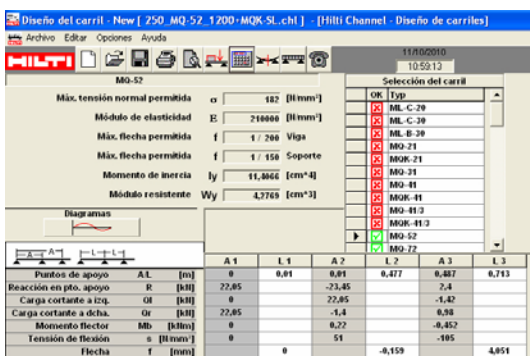
Cálculo de soportes con el software Hilti Channel.
