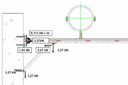
Fuerzas de reacción en los soportes.
