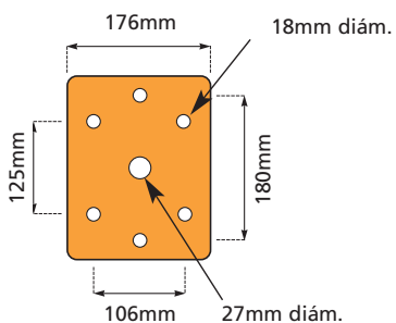
Planta típica de placa final
