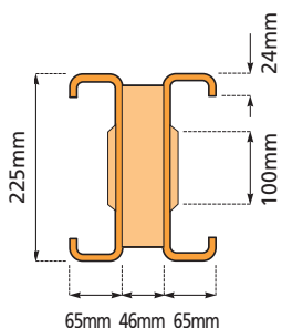
Sección típica
