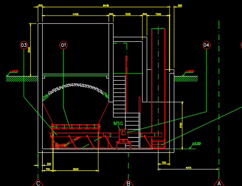
Schnitt D-D
