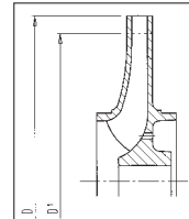
Réduction du diamètre externe du rotor pour pompe centrifuge par tournage.
