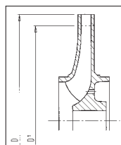
Réduction du diamètre extérieur du rouet pour pompe centrifuge par tournage.
