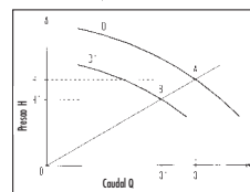
Diagrama para determinar o diâmetro de torneamento.
