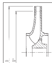
Reducción con torneado del diámetro exterior del rodetes para bomba centrífuga.
