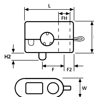
Abrazaderas Retenedoras KK
