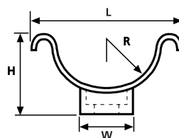
Clips Tipo Cuna C1 - 3
