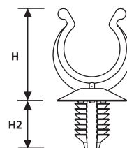
PC-Clip con fijación de cabeza de abeto
