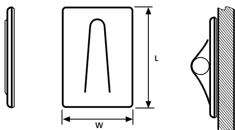
Clip Adhesivo Serie SAC
