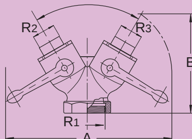
BIFURCACIÓN 70 mm.
