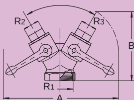
BIFURCACIÓN 45 mm.
