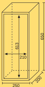
MARCO FIJO EXT 6-12 kg REF. EXTMF6
