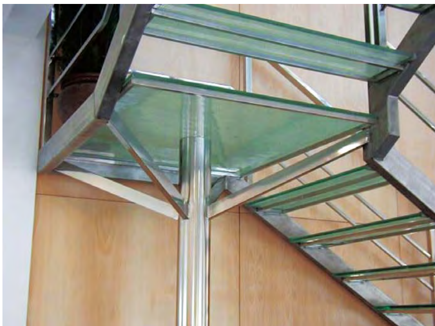
Modelo 1: Soporte en acero Inox para escalera con peldaños de cristal
