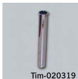
Inlet extensión dimensions: 200 mm 300 mm material: chrome plated brass
