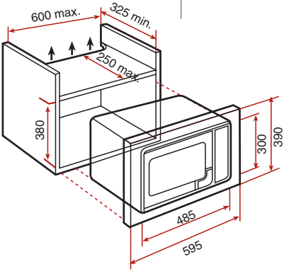
TMW 18 BIH TMW 18 BI
