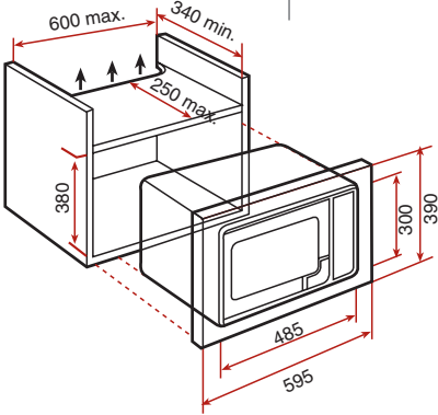
TMW 22 BIT TMW 22 BIS TMW 22 BI
