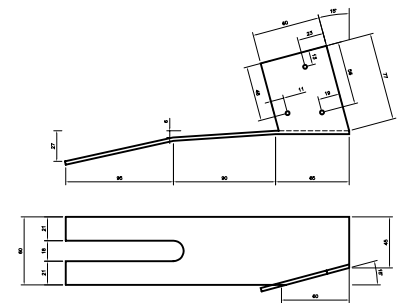
CHAPA DE ACERO DE 3 mm
