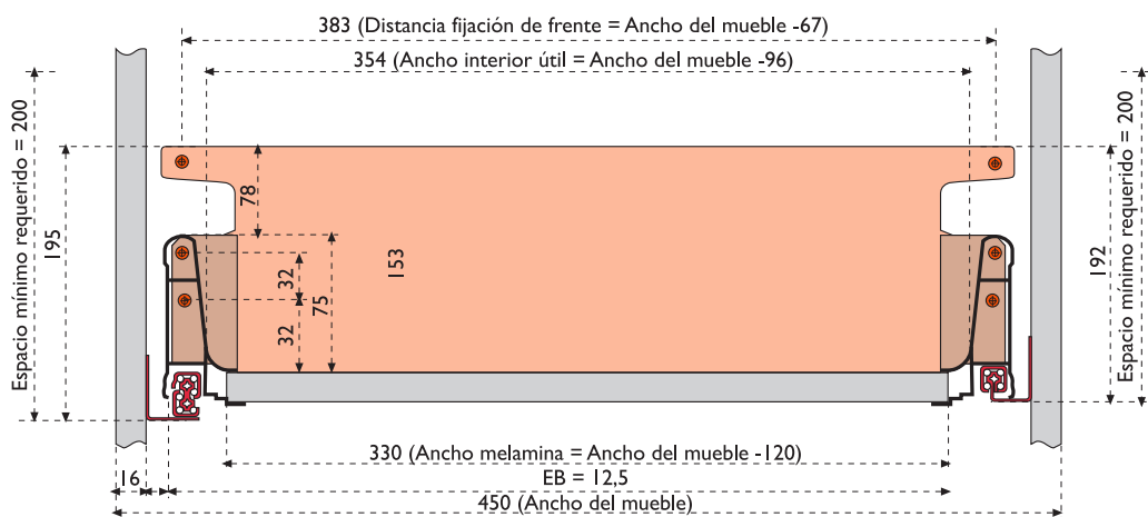
Figura de la izquierda: Alutec con Quadro V6 de extracción total Figura de la derecha: con Quadro de extracción parcial
