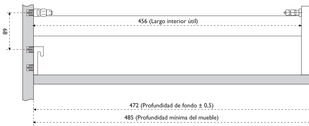
Figura de la izquierda: Alutec con Quadro V6 de extracción total Figura de la derecha: con Quadro de extracción parcial
