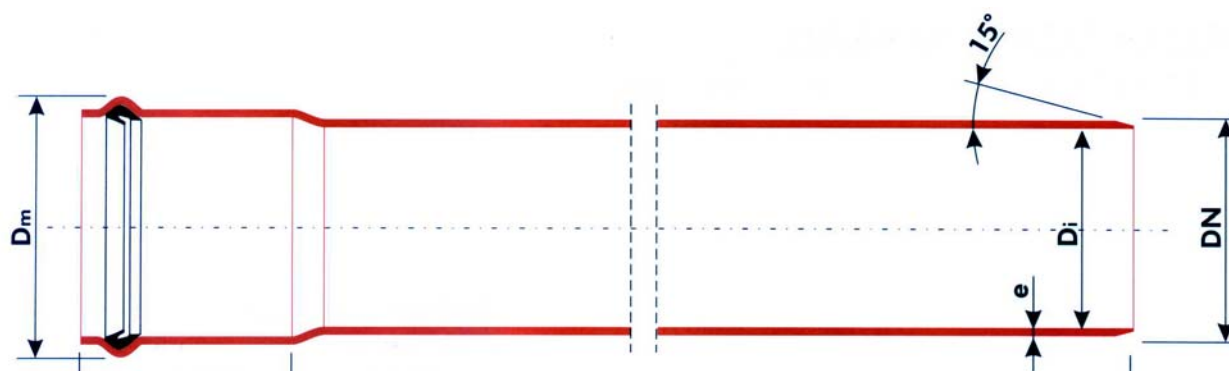
SERIE SN 4 NORMAS 1401 Y 1456 (PN6)
