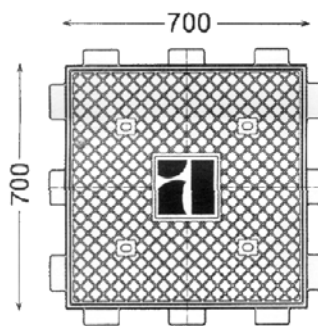
Modelo TM-2 Nodular B-125
