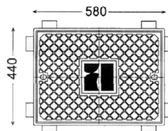
Modelo TM-1 Nodular B-125
