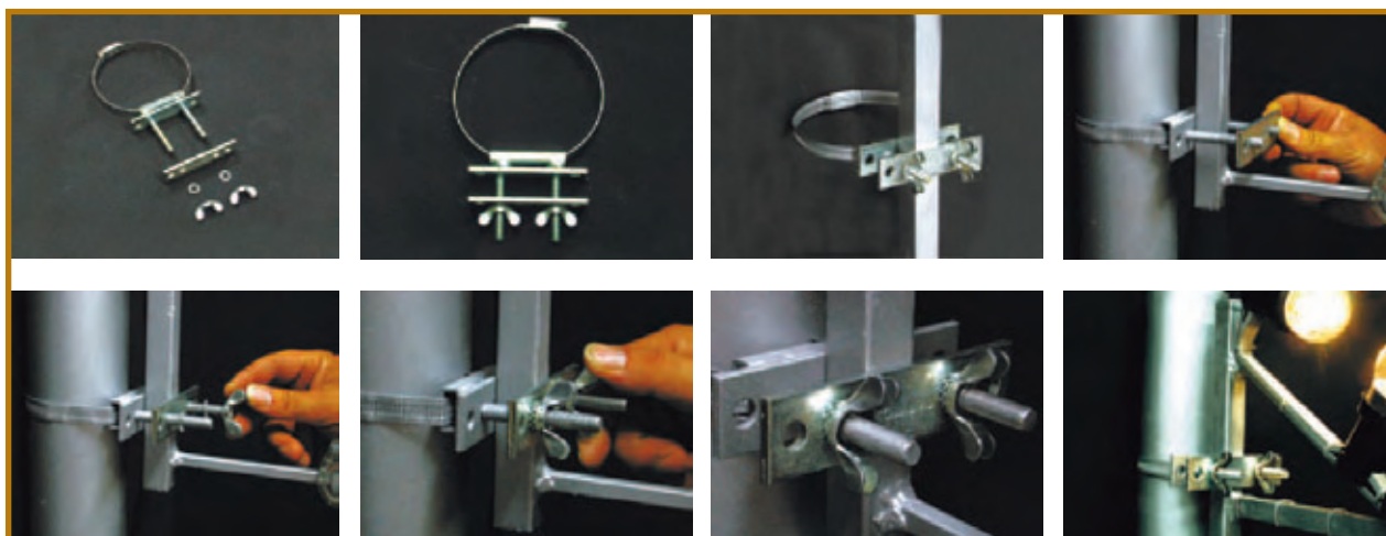
REF. 0307701 SUJECION FIGURA / FIXAÇ O FIGURA
