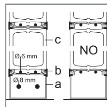
a perfil en "U" b perfil c bloques de cristal
