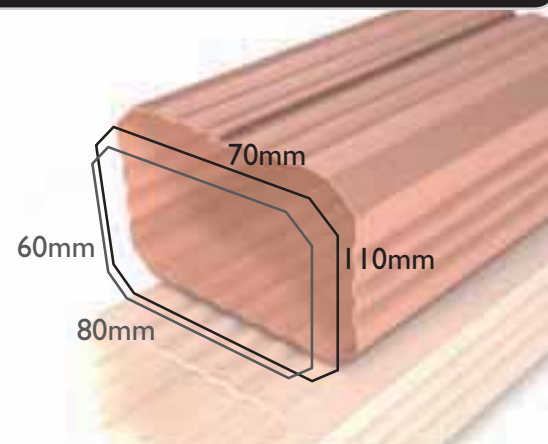
Bajante Rectangular
