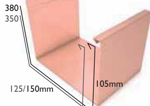
Canalón Industrial
