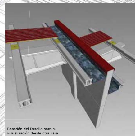
Vista de Detalle constructivo de cubierta sobre cerramiento y pilar medianero con salto entre naves,
