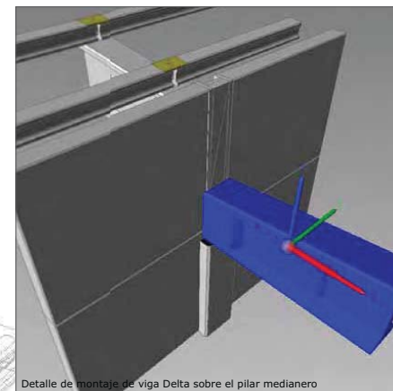
Detalle de montaje de viga Delta sobre el pilar medianero
