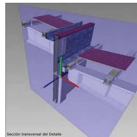
Sección transversal del Detalle
