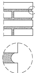
Junta redondeada o fratasada
