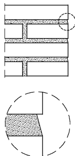
Figura 2: Tipología de acabado de juntas en fábricas vistas.
