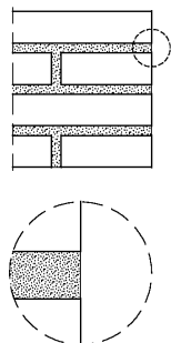
Figura 2: Tipología de acabado de juntas en fábricas vistas.
